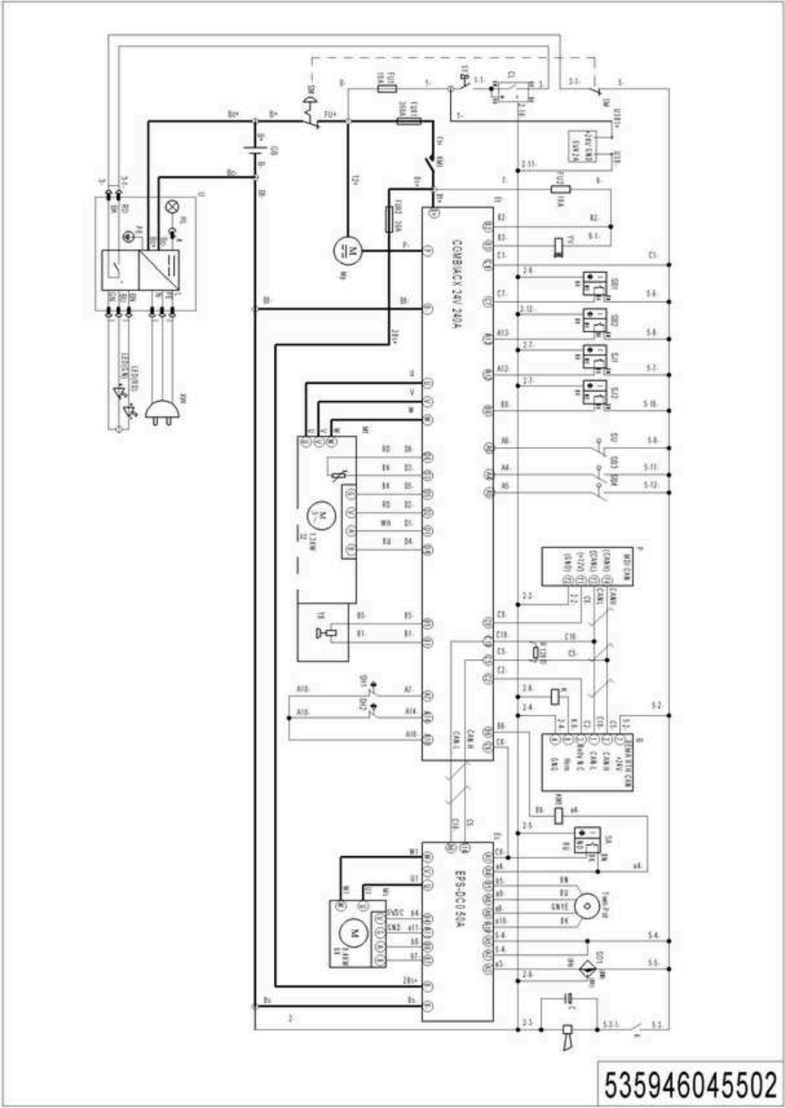
03 Схема электрической цепи (усилитель рулевого управления)
