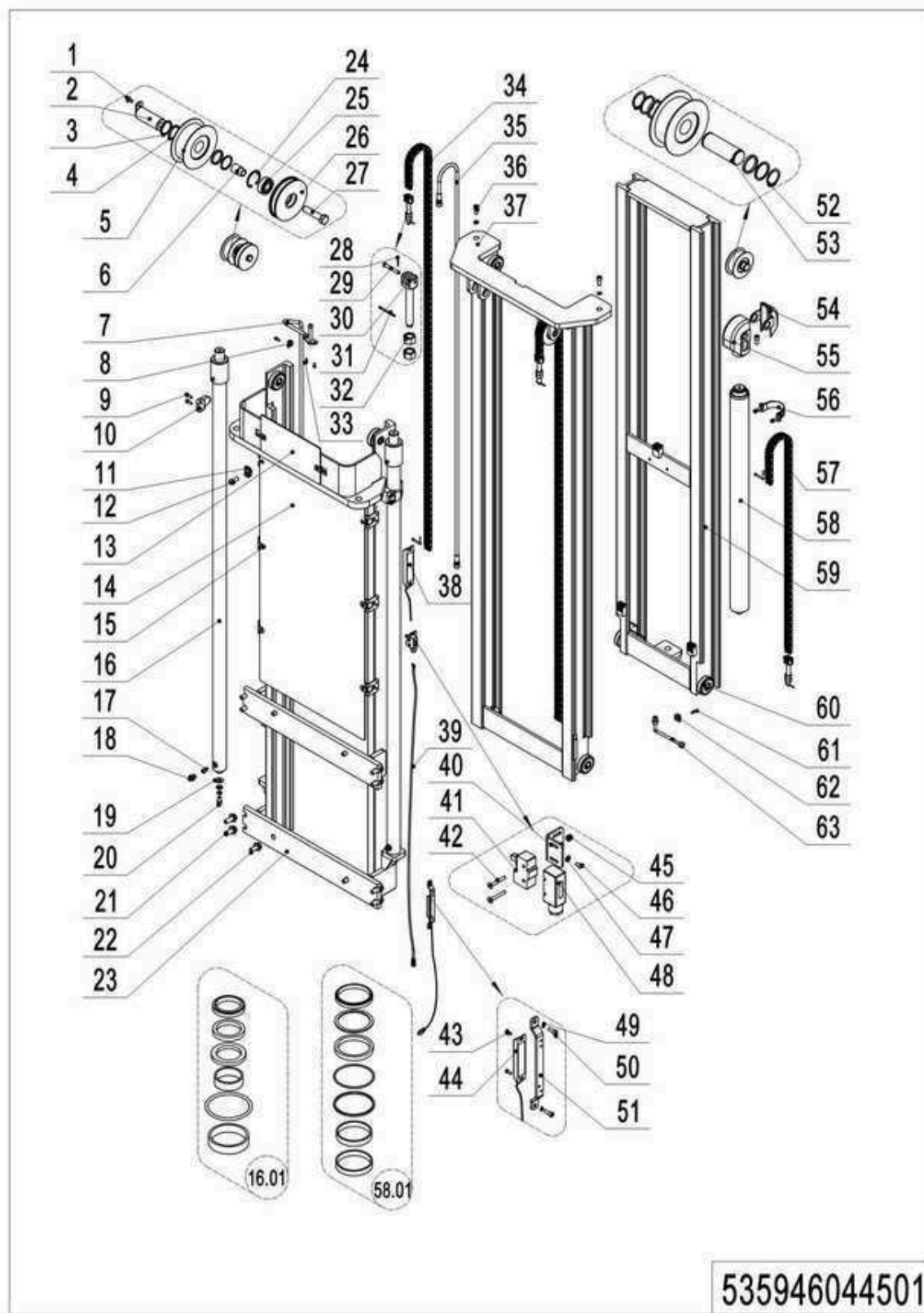
04 Тройной мачтовый подъемник с полным свободным подъемом (535946044501)
