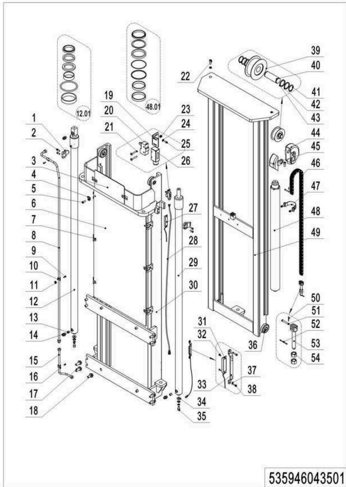
02 Двухступенчатый мачтовый механизм полного свободного подъема (535946043501)
