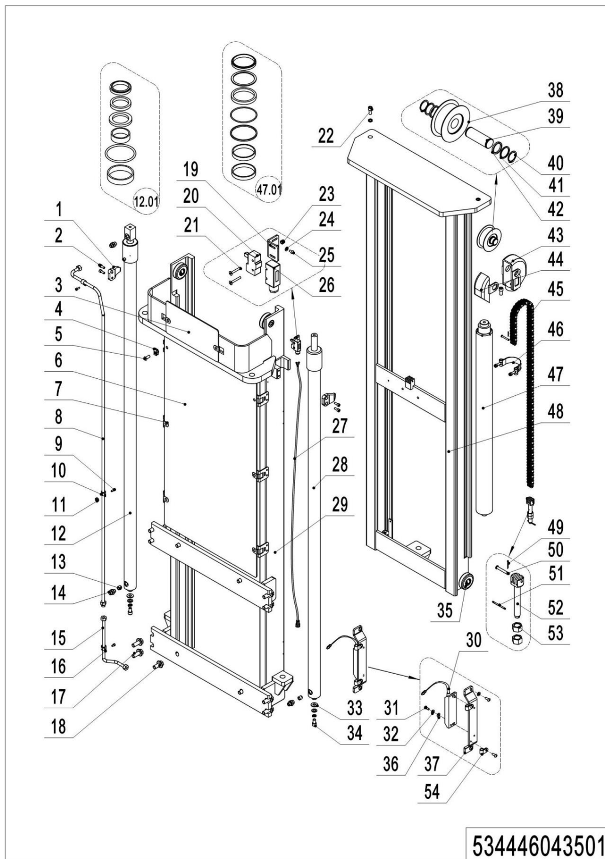
02 Двухступенчатый мачтовый механизм полного свободного подъема (534446043501)
