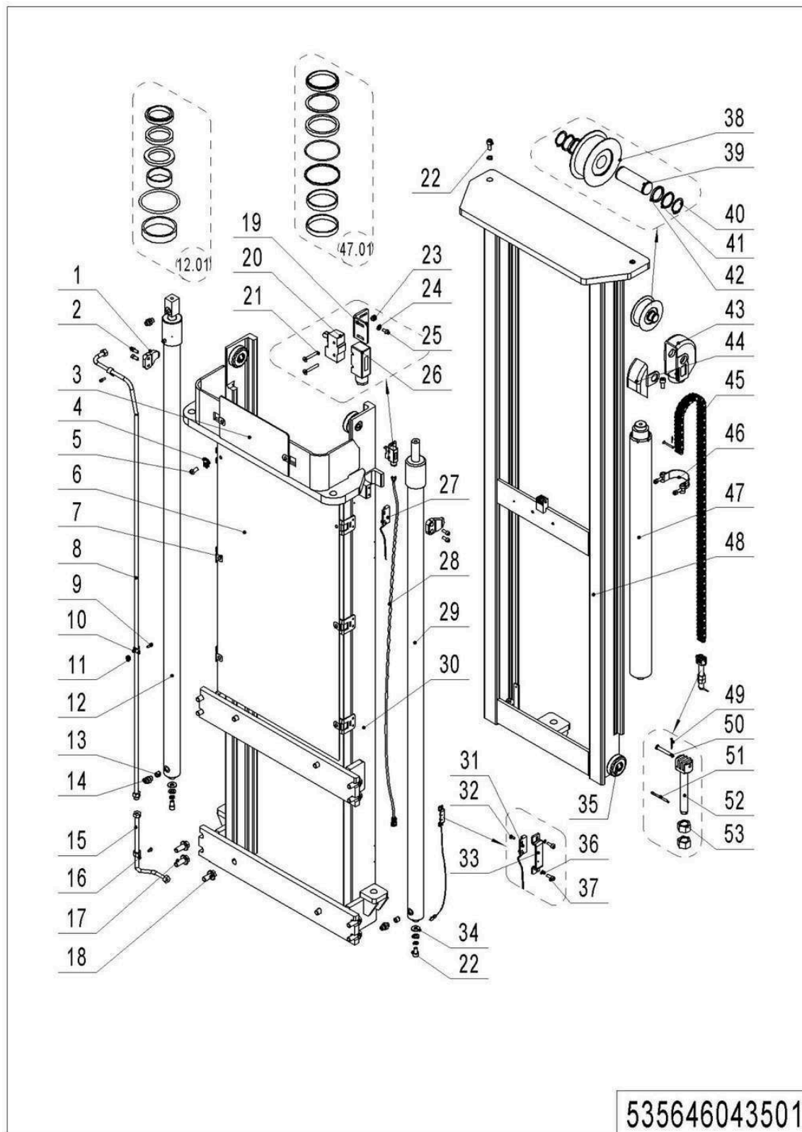
02 Двухступенчатый мачтовый механизм полного свободного подъема (535646043501)
