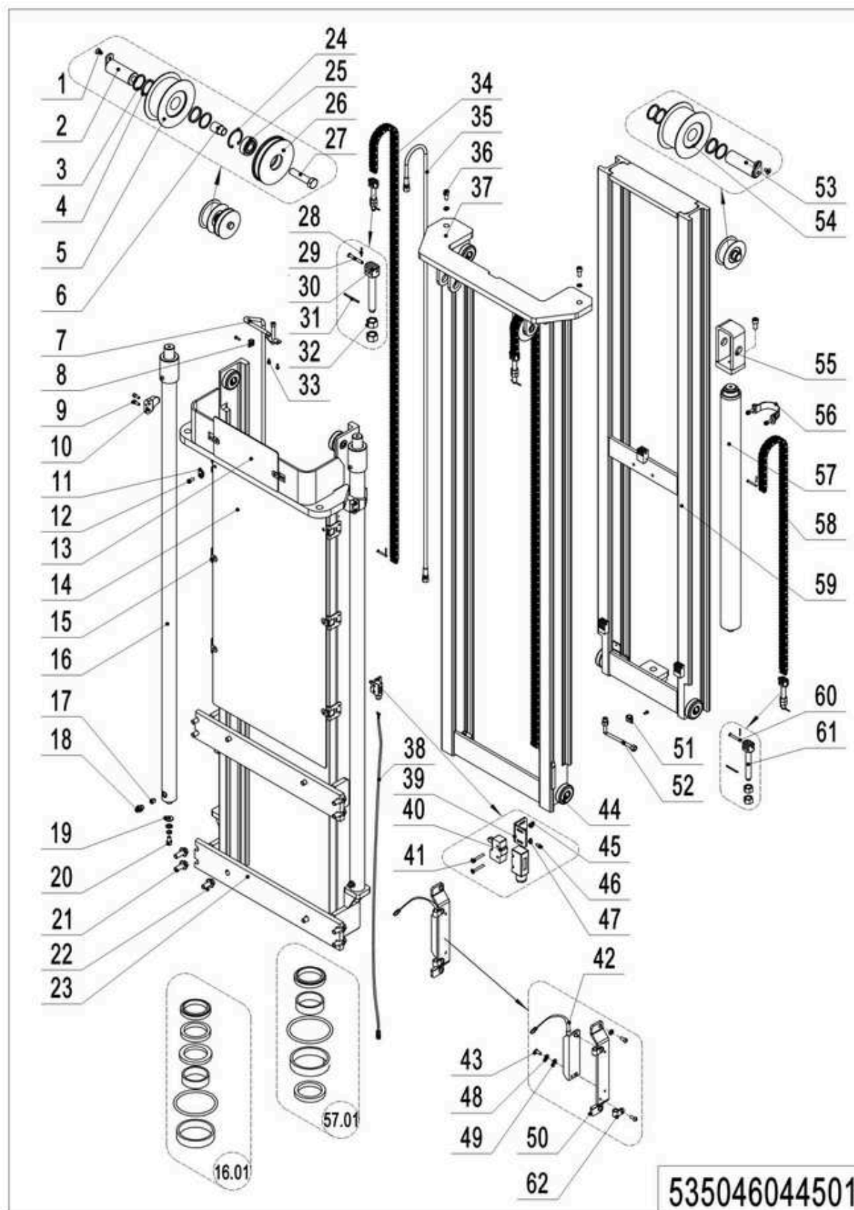
04 Тройной мачтовый подъемник с полным свободным подъемом (535046044501)
