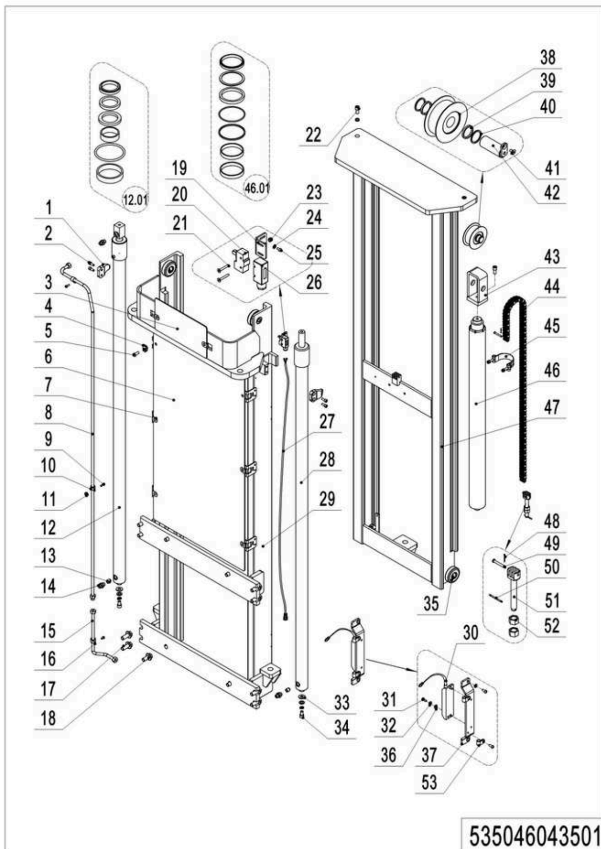
02 Двухступенчатый мачтовый механизм полного свободного подъема (535046043501)
