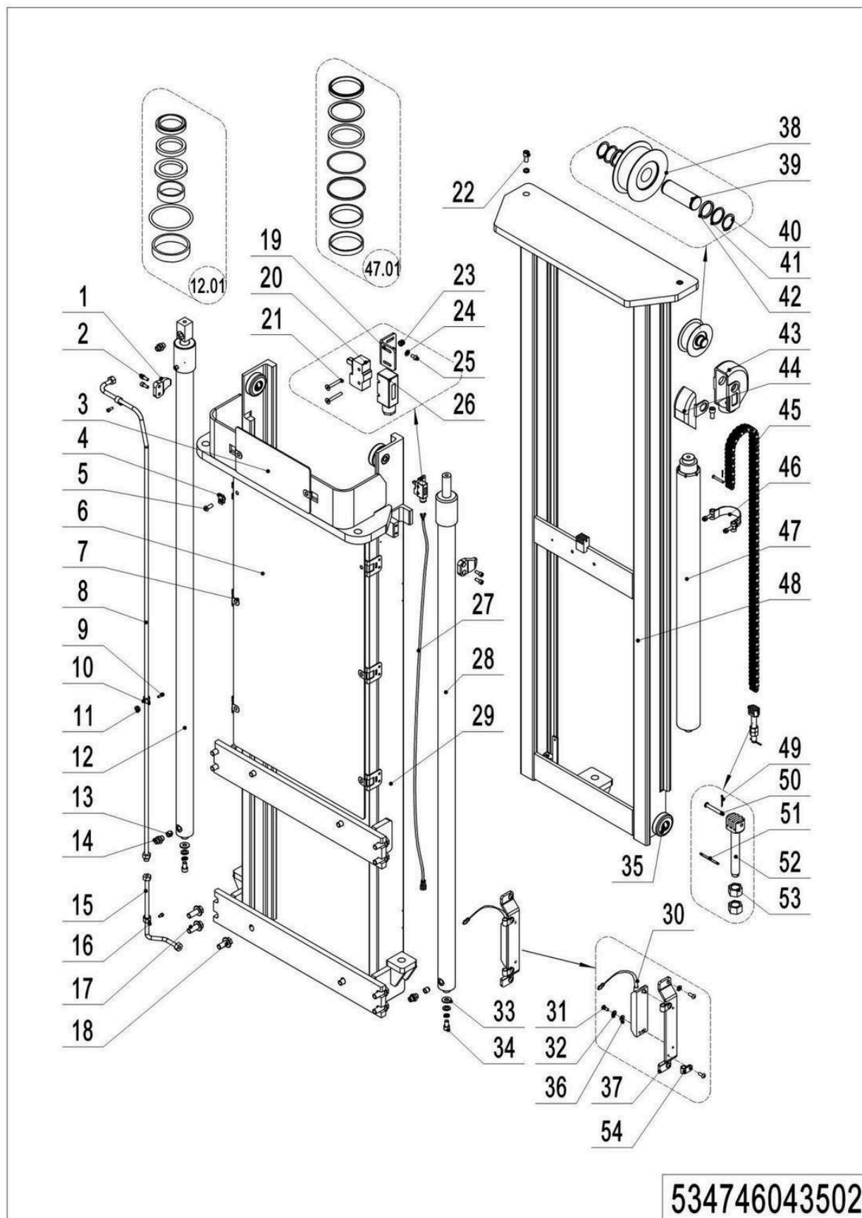
02 Двухступенчатый мачтовый механизм полного свободного подъема (534746043502)
