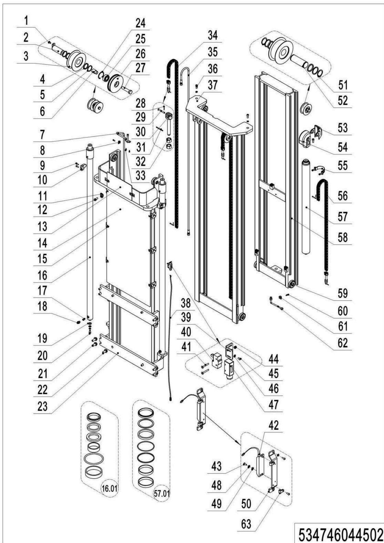
04 Тройной мачтовой подъемник с полным свободным подъемом (534746044502)
