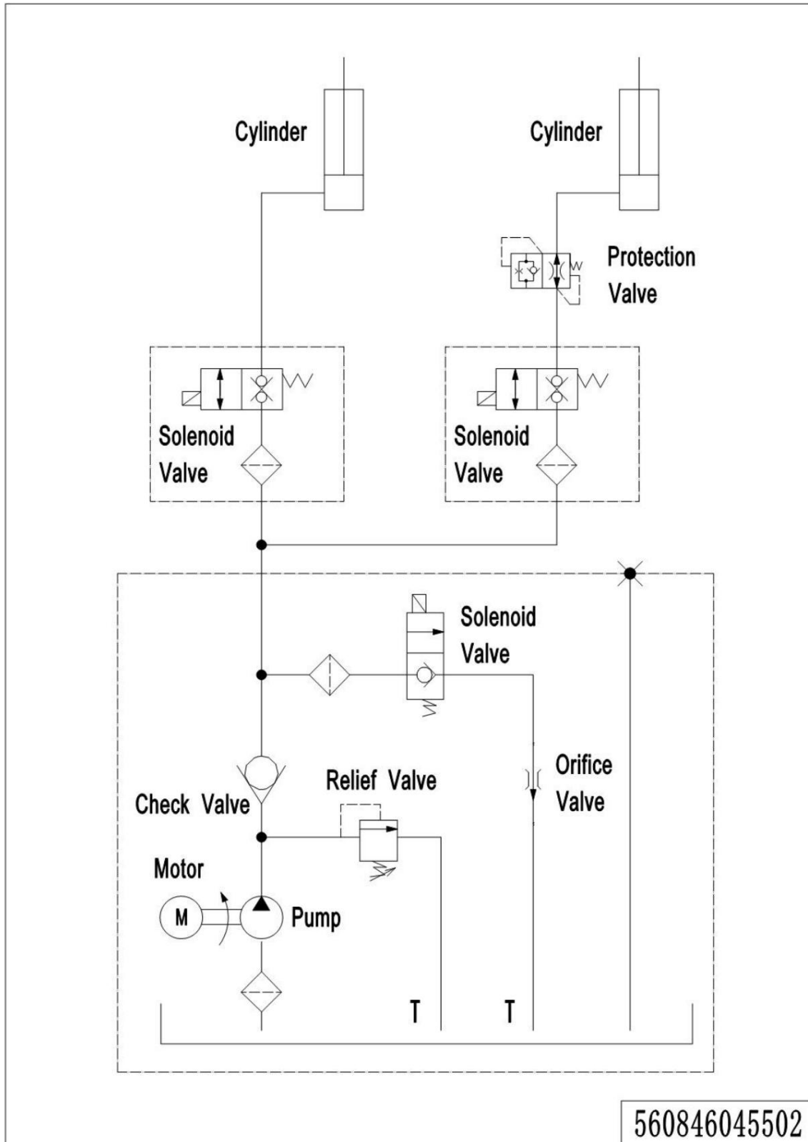
01 Схема гидравлической цепи (560846045502)
