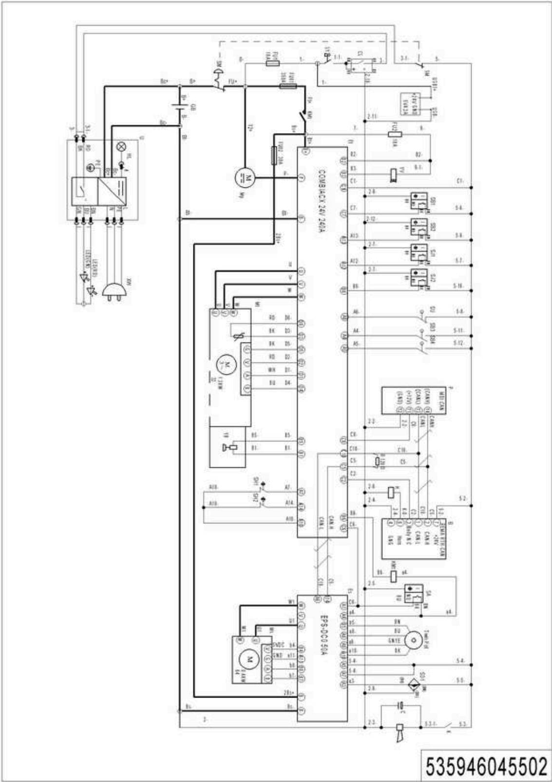
01 Схема электрической цепи
