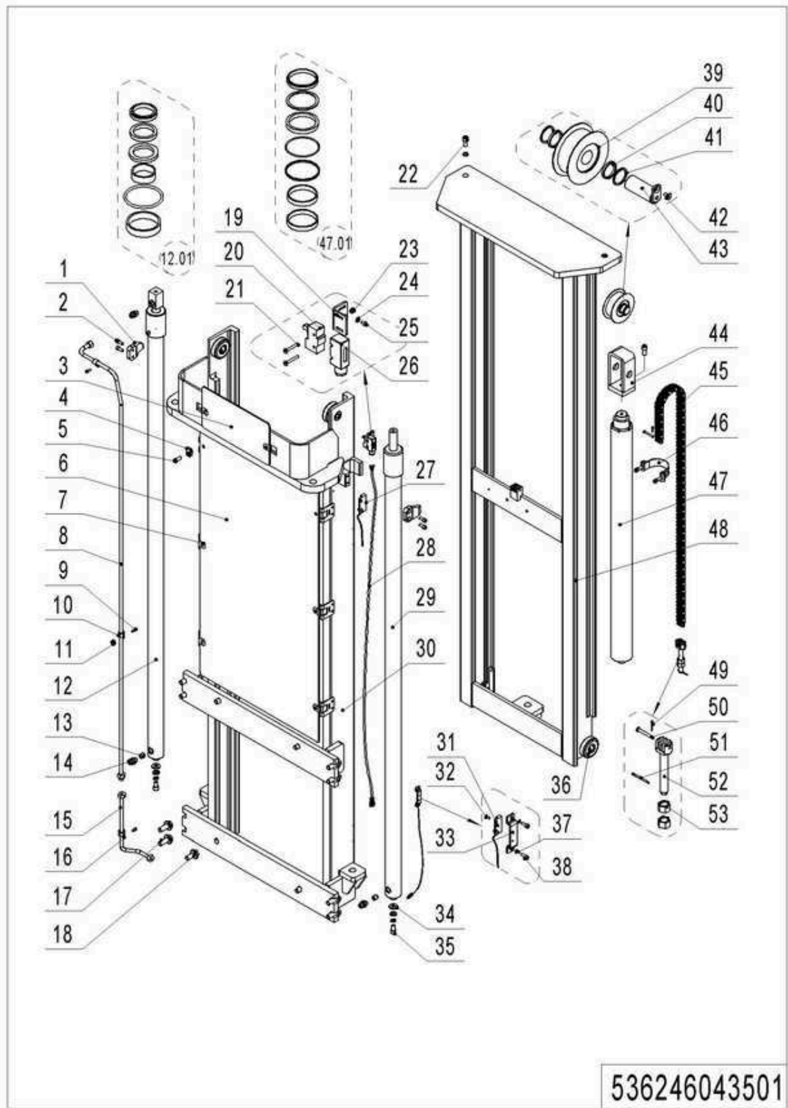
02 Двухступенчатый мачтовый механизм полного свободного подъема (536246043501)
