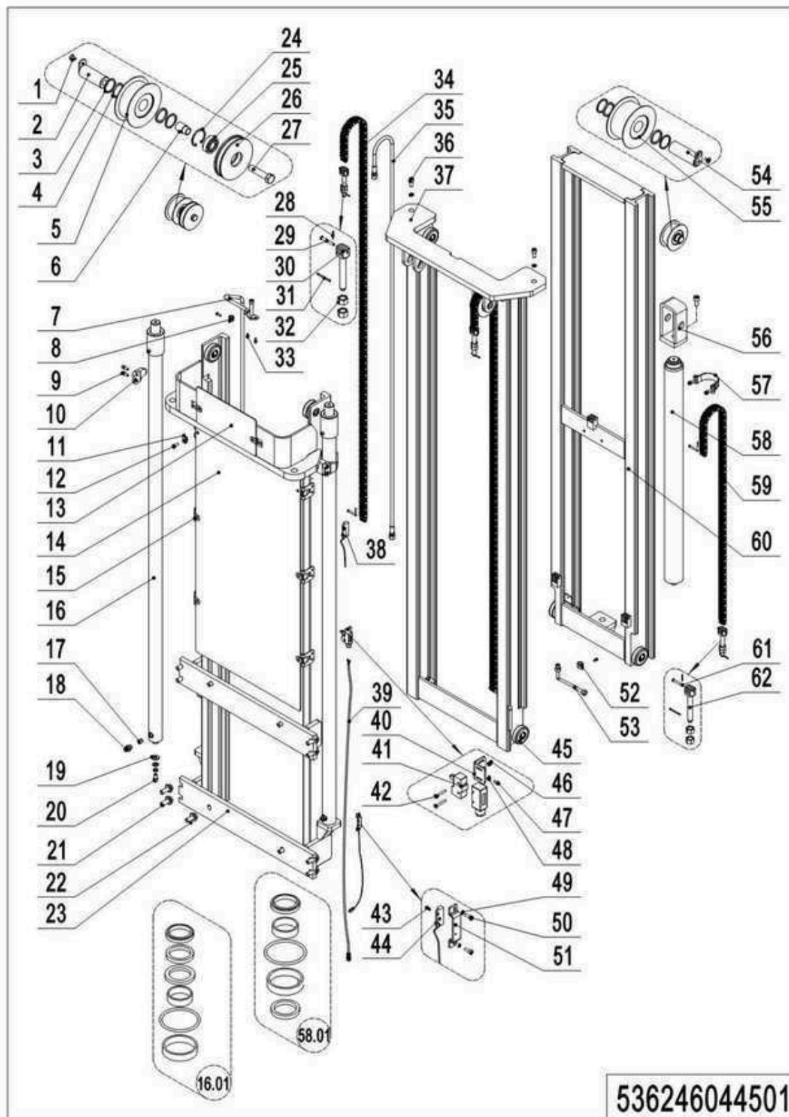
04 Тройной мачтовый подъемник с полным свободным подъемом (536246044501)
