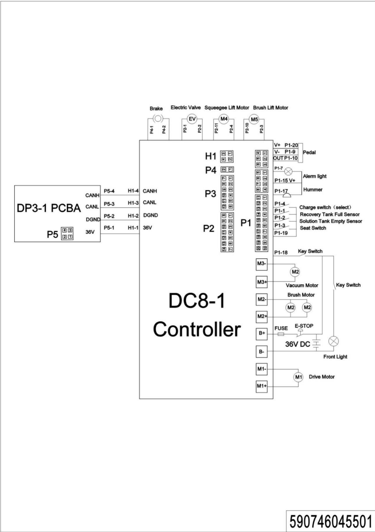
01 Схема электрической цепи (свинцово-кислотный аккумулятор) (590746045501)
