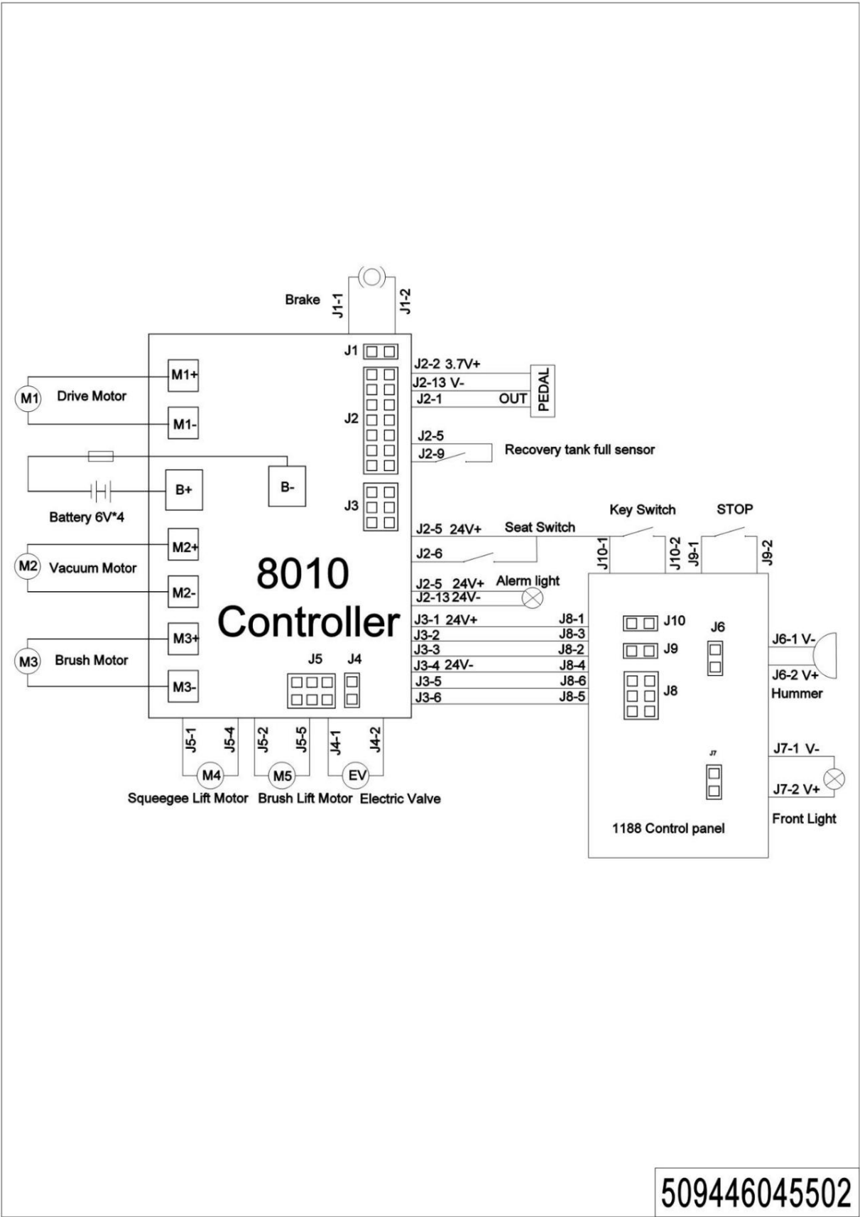
01 Схема электрической цепи (свинцово-кислотный аккумулятор) (509446045502)
