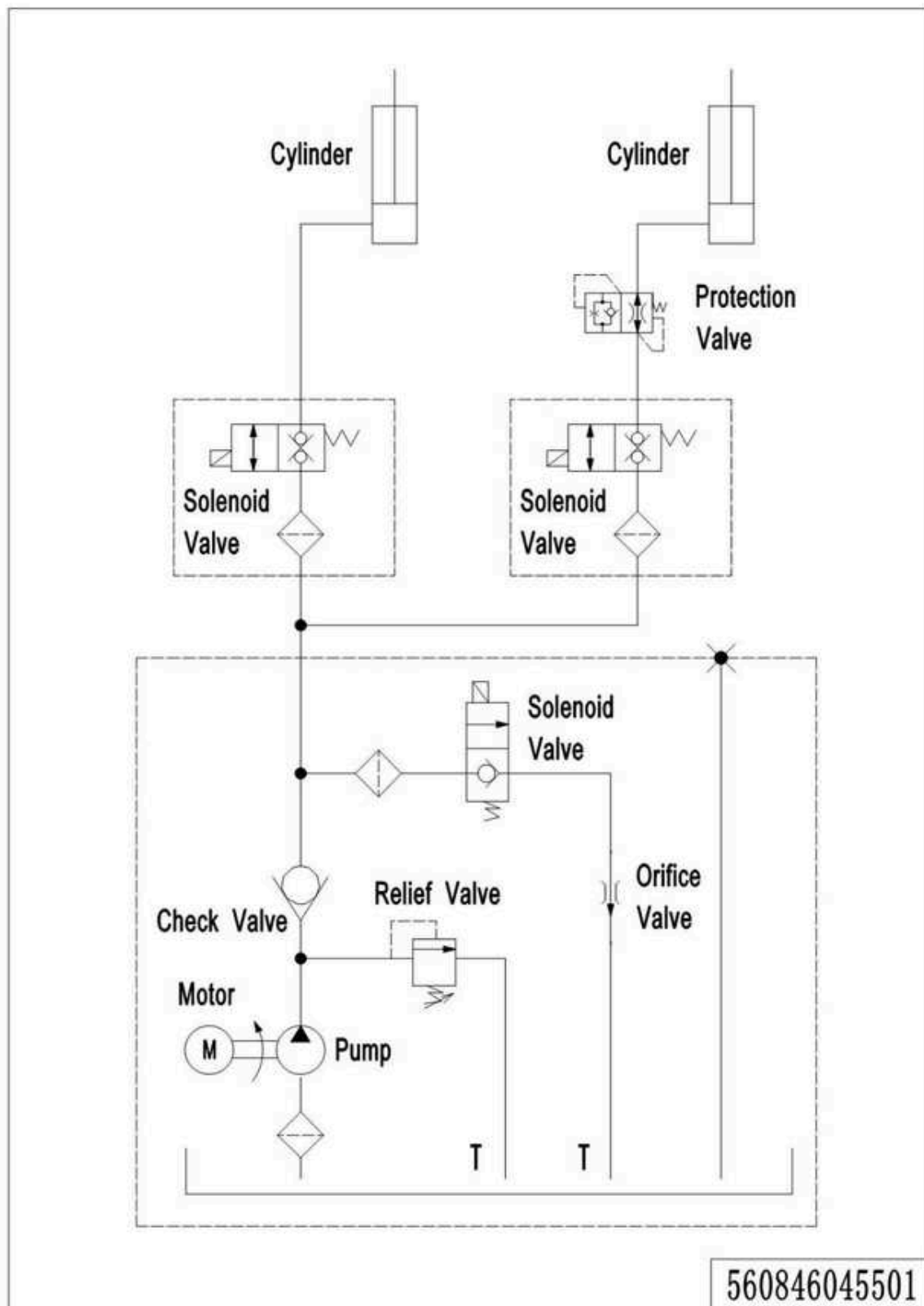
01 Схема гидравлической цепи (560846045501)
